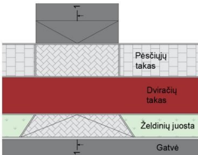
Pjūvis 1-1
