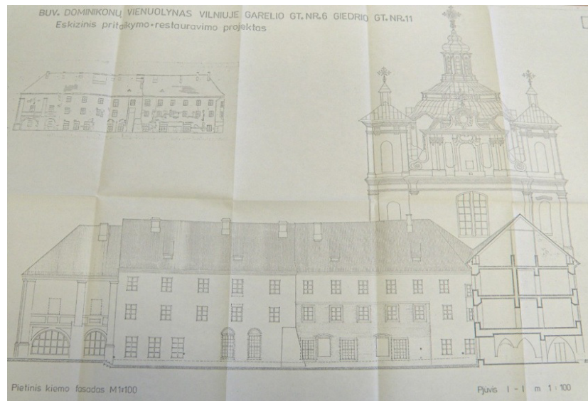
2.14 pav. Pietinio kiemo korpuso „B“ fasadas ( Kultūros vertybių... 2014 )
