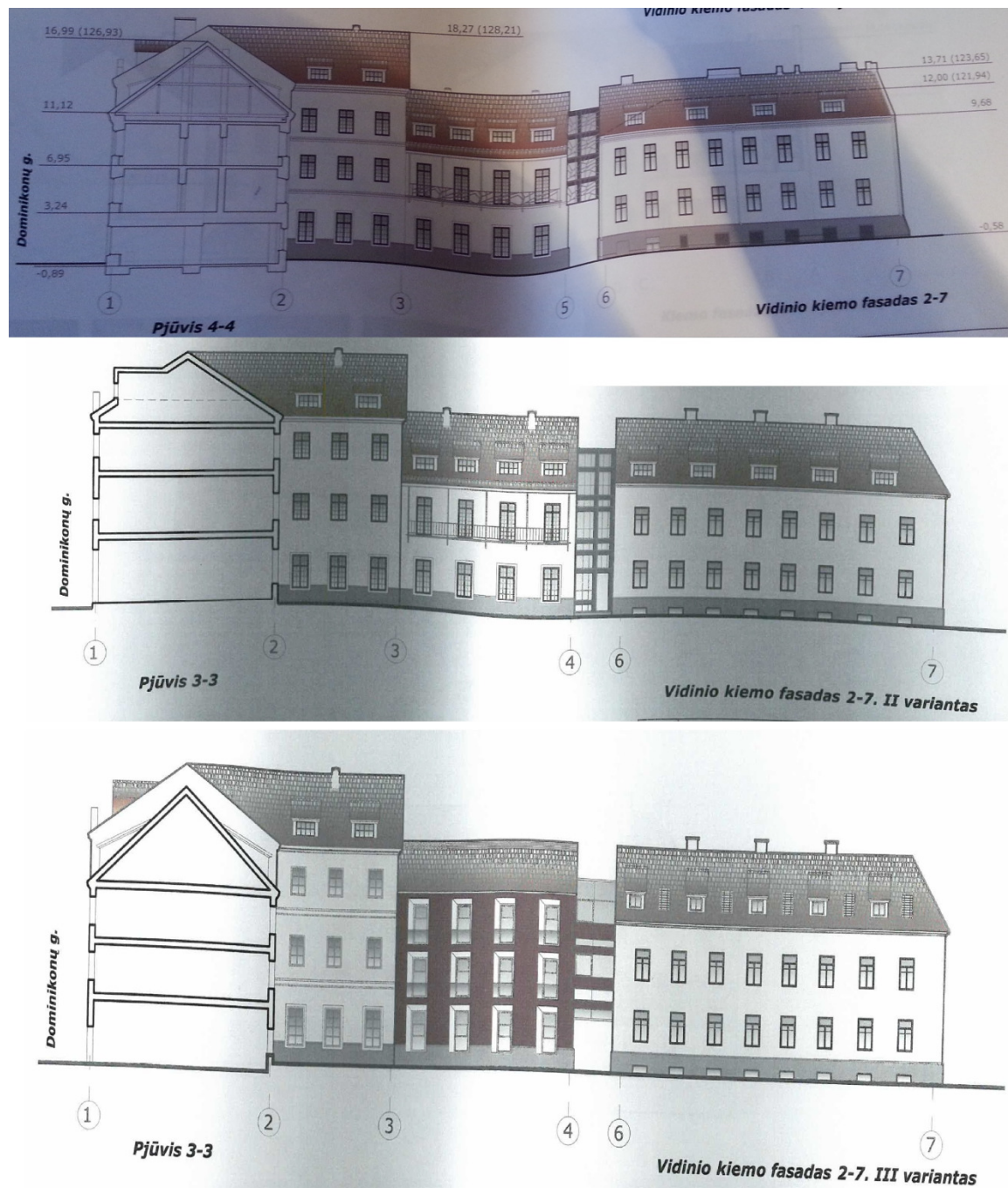
5.10 pav. Vidinio kiemo fasado tarp ašių 2-7 išklotinės ( Kliobavičiūtė et al. 2008 )
