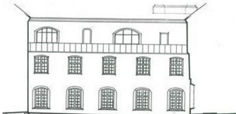
2.10 pav. Keturkampio kiemo vakarinio fasado išklotinė ( Kultūros vertybių... 2014 )
