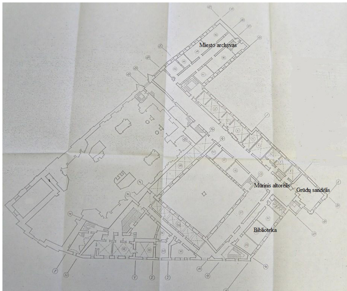
2.3 pav. Antro aukšto patalpų išdėstymas ( Kultūros vertybių... 2014 )
