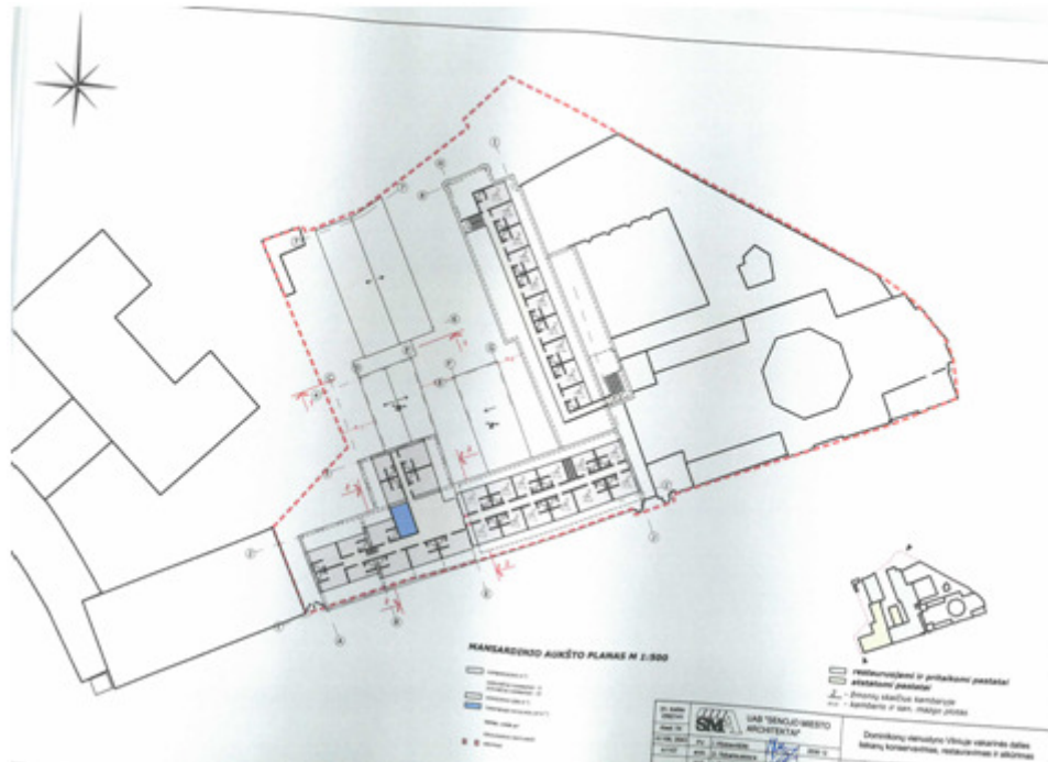
5.21 pav. Mansardinio aukšto planas – II variantas ( Kliobavičiūtė et al. 2008 )
