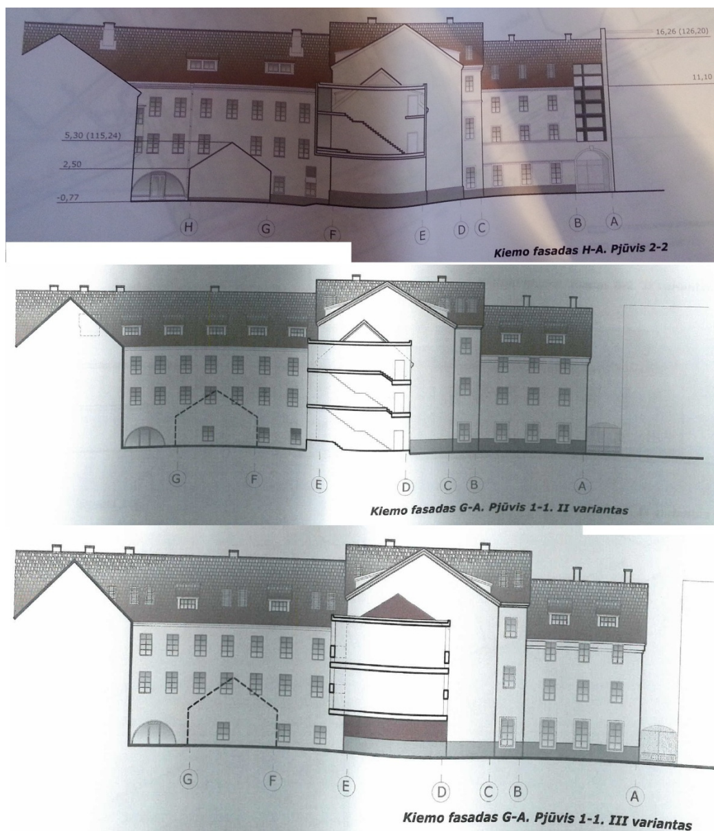
5.9 pav. Kienio fasado tarp ašių H-A ir G-A išklotinės ( Kliobavičiūtė et al. 2008 )
