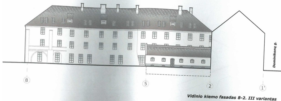
5.11 pav. Vidinio kiemo fasado tarp ašių 4-2 ir 8-2 išklotinės (Kliobavičiūtė et al. 2008)
